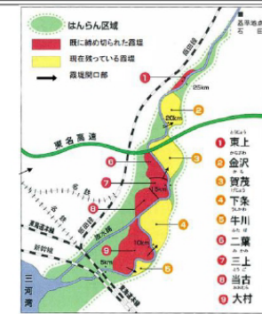
現在の霞堤の開閉状況 出典: 国土交通省中部地方整備局豊橋河川事務所『豊川の霞堤』(2013.10.31)
